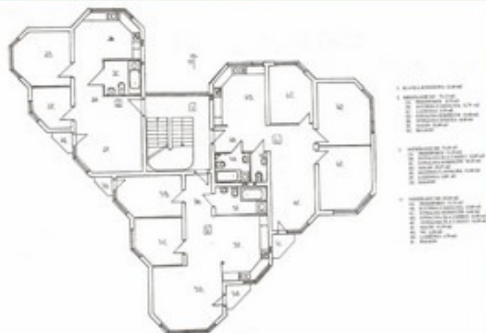
RZUT I,II PIĘTRA
